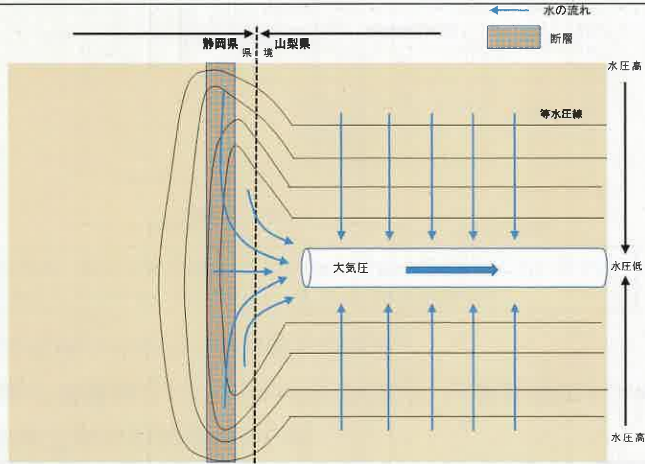
【図2:断層がある場合の周辺からトンネルに水が引き込まれる概念図(トンネルを上から見た場合)】
